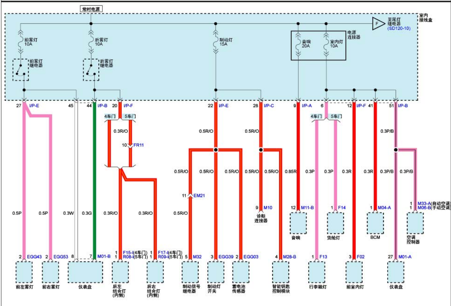
室内保险丝分布(9)
